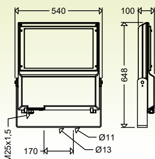
Swivel range
